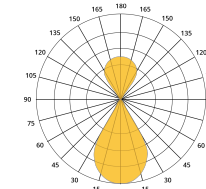
Uneven Distribution
