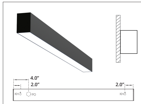
WALL FLUSH
